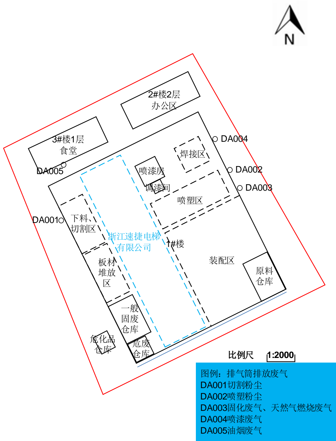
附图 4 全厂总平面布置示意图
